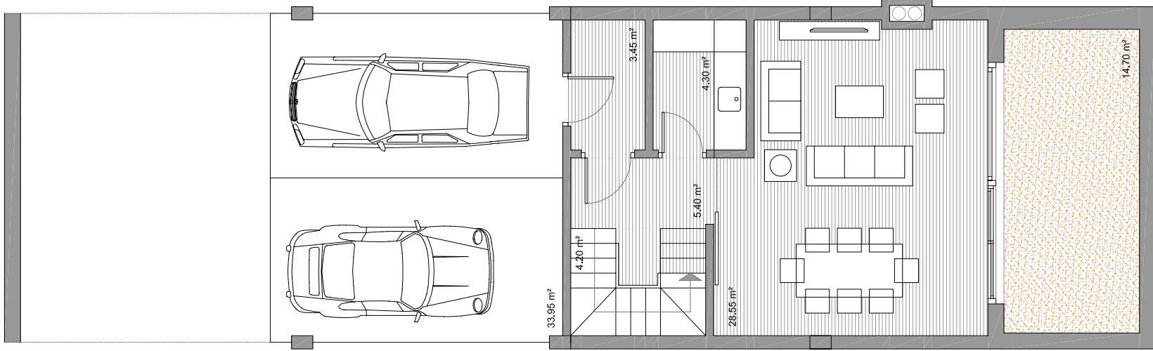
PLANTA SÓTANO
