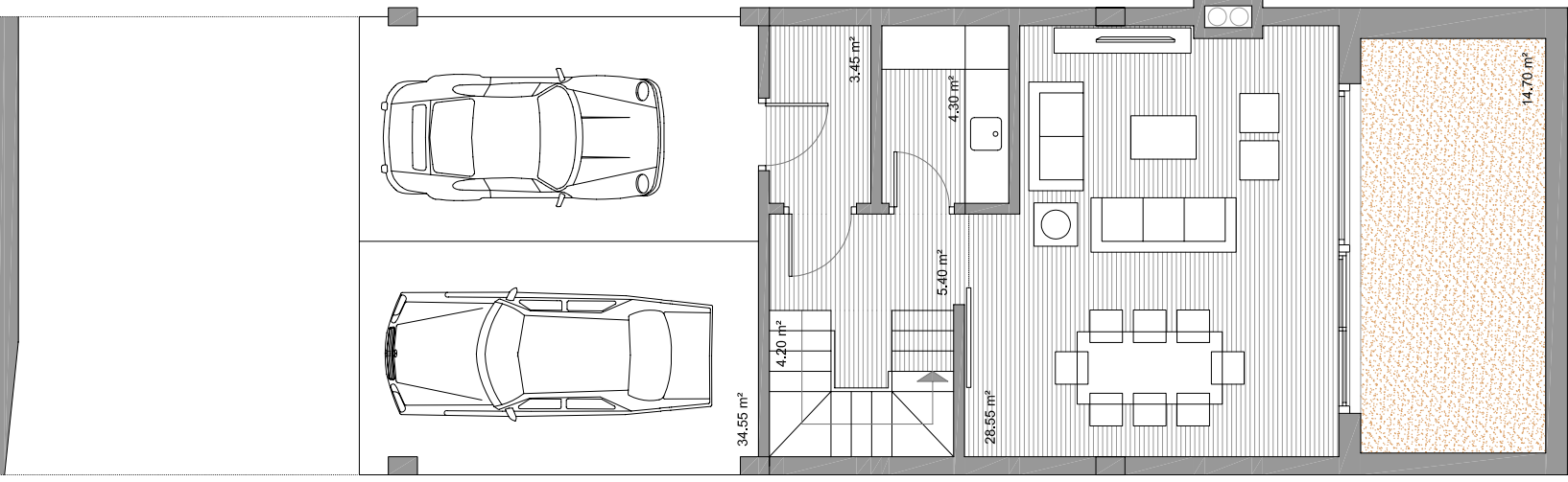
PLANTA SÓTANO
