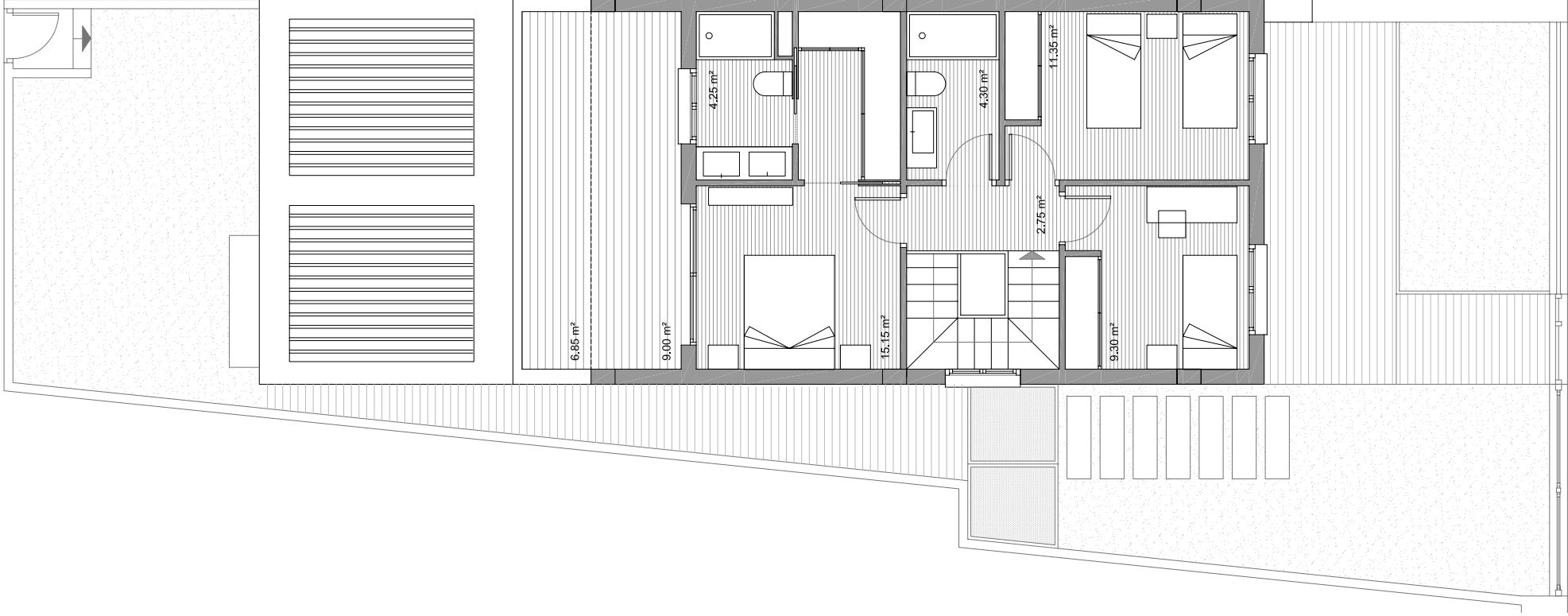
PLANTA PRIMERA
