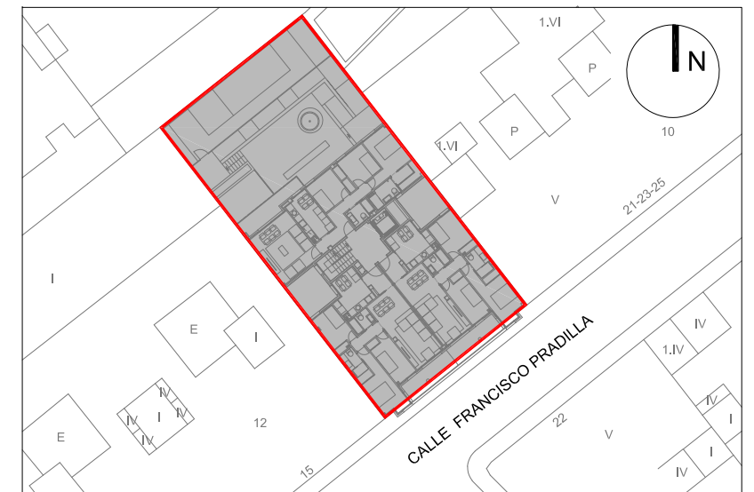
PLANTA SOTANO -1
